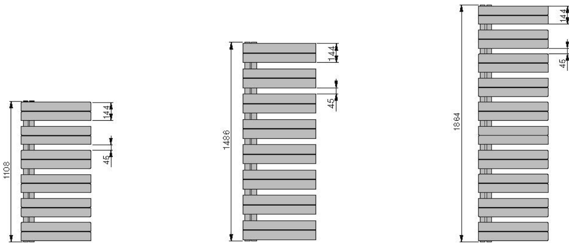
Vorderansicht ROI-120-060
