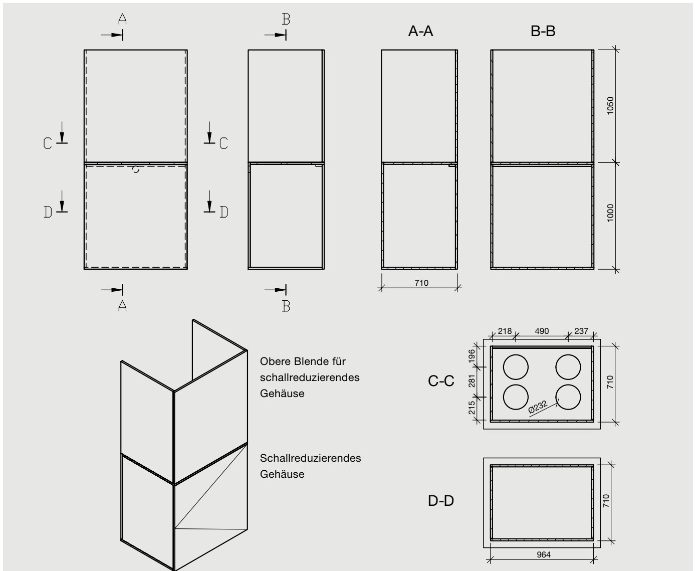
Zehnder ComfoAir Q600 ST mit schallreduzierenden Gehäuse
