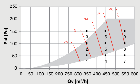
Zehnder ComfoAir Q600 ST mit schallreduzierenden Gehäuse
